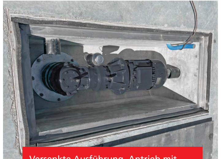
Versenkte Ausführung, Antrieb mit Winkelgetriebe und Motor
