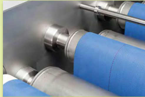
Presswalzen auf stehenden Wellen mit gekapselten Walzenlagern gelagert – keine Wechselbiegung
