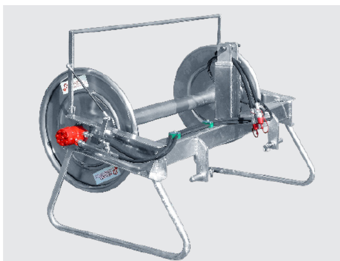
Schlauchhaspel SHW 400 mit Hydraulik-Antrieb und Dreipunktaufhängung
